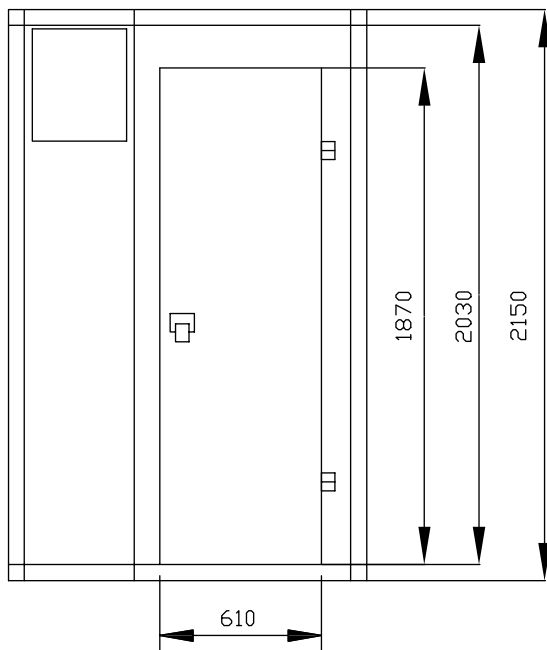
Zij aanzicht
